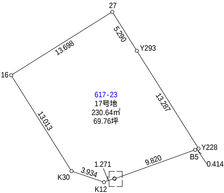
拡大図 S=1/20
